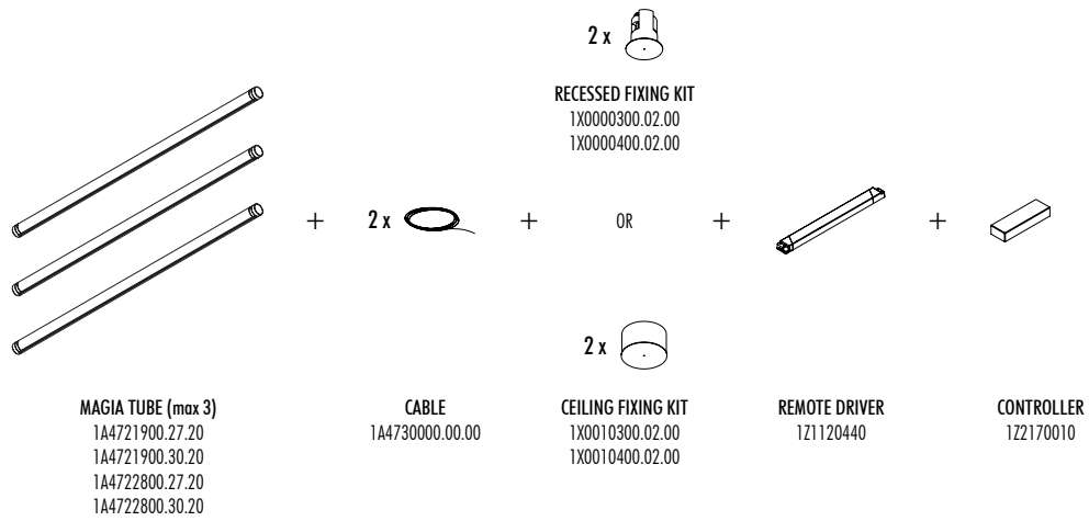
ESEMPIO DI INSTALLAZIONE MULTIPLA CON KIT FISSAGGIO DA INCASSO O A SOFFITTO / EXAMPLE OF MULTIPLE INSTALLATION WITH RECESSED FIXING KIT OR CEILING FIXING KIT
