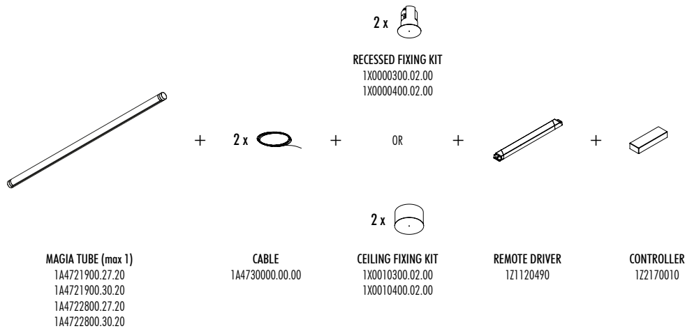
ESEMPIO DI INSTALLAZIONE SINGOLA CON KIT FISSAGGIO DA INCASSO O A SOFFITTO / EXAMPLE OF SINGLE INSTALLATION WITH RECESSED FIXING KIT OR CEILING FIXING KIT
