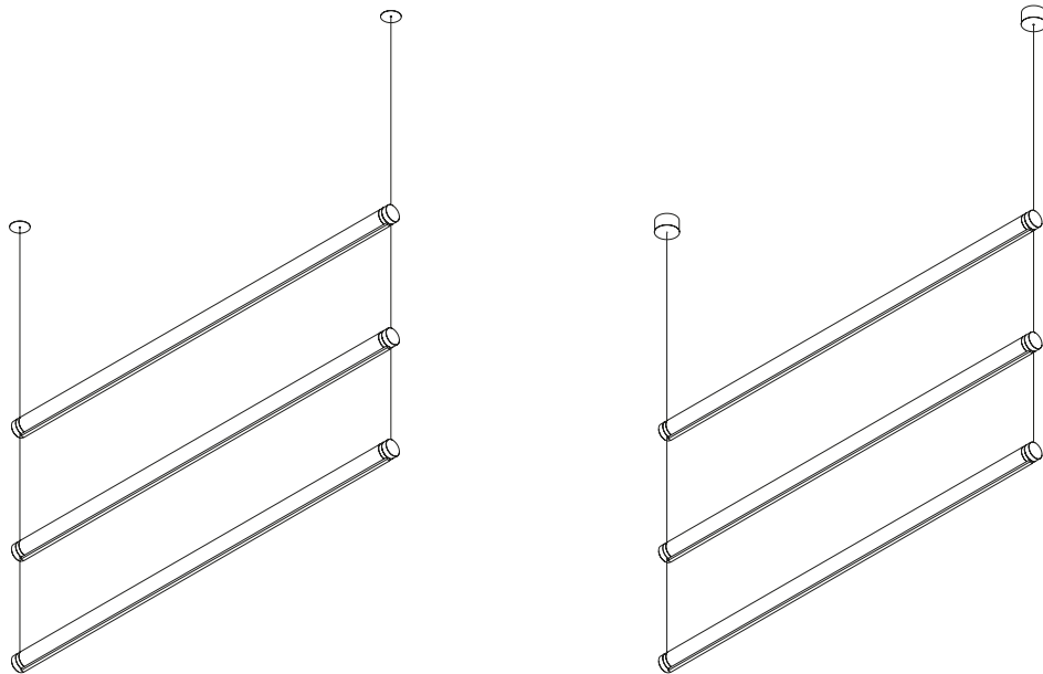
ESEMPIO DI INSTALLAZIONE MULTIPLA CON KIT FISSAGGIO DA INCASSO O A SOFFITTO / EXAMPLE OF MULTIPLE INSTALLATION WITH RECESSED FIXING KIT OR CEILING FIXING KIT
